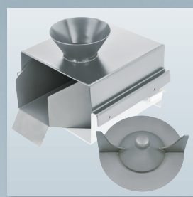
Насадка для протирания с лотком, нержавеющая сталь 104 036 000 Внимание: основное универсальное устройство не включено в комплект поставки Лопасть для протирочного барабана, нержавеющая сталь 100, 200, 300 104 075 000
