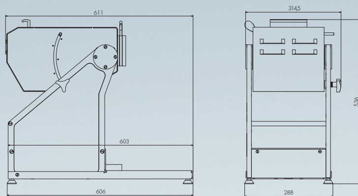
M 4 Многоцелевая кухонная машина
