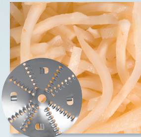
Дисковый нож для шинковки, нержавеющая сталь, ручная заточка 6 мм 561 000 0372* 9 мм 561 000 0373
