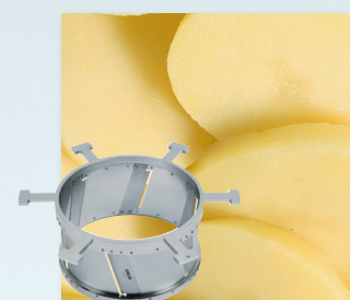
Цилиндр для нарезки, нержавеющая сталь 1,5 мм, зубчатый, с 6 ножами 548 100 3815 2 мм, зубчатый, с 6 ножами 548 100 3820 2,5 мм, зубчатый, с 6 ножами 548 100 3825 4 мм, гладкий с 6 ножами 548 100 3840 6 мм, гладкий с 6 ножами 548 100 3860
