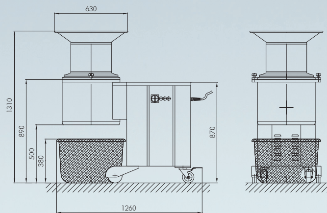
G 450 Универсальная овощерезка
